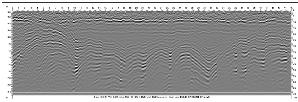
Figur 24 - Georadarprofil. Profilen representerer et digitalt tverrsnitt gjennom jorda. De øverste 30 cm er matjord. Overgangen mellom matjorden og den naturlige undergrunnen er markert med en rekke lineære refleksjoner som strekker seg horisontalt gjennom datasettet. De ondulerende linjene som kan observeres i bunnen av datasettet representerer løsmasser fra et uttørket elveleie. Illustrasjon: NIKU.
