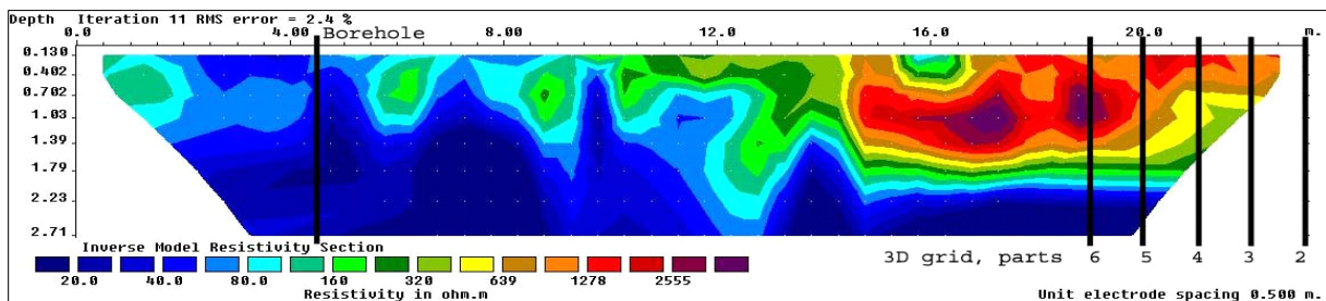
Figur 17 - Digital profil basert på ERT-målinger ved en arkeologisk utgravning i Nedre Langgate i Tønsberg i 2009. Blå områder tyder på tette lag med høyt vanninnhold og høye konsentrasjoner av redusert jern, mens oransje og røde områder indikerer porøse, noe tørrere områder med lavere konsentrasjoner av redusert jern (Bergersen et al. 2008).
