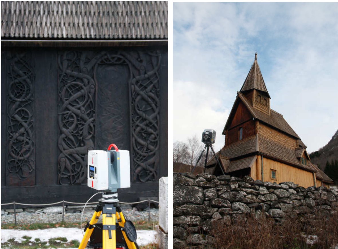
Figur 1 - Leica HDS6000 fasebasert laserskanner (til venstre) og Trimble GS200 pulsbasert laserskanner (til høyre). Foto: Knut Paasche, NIKU
