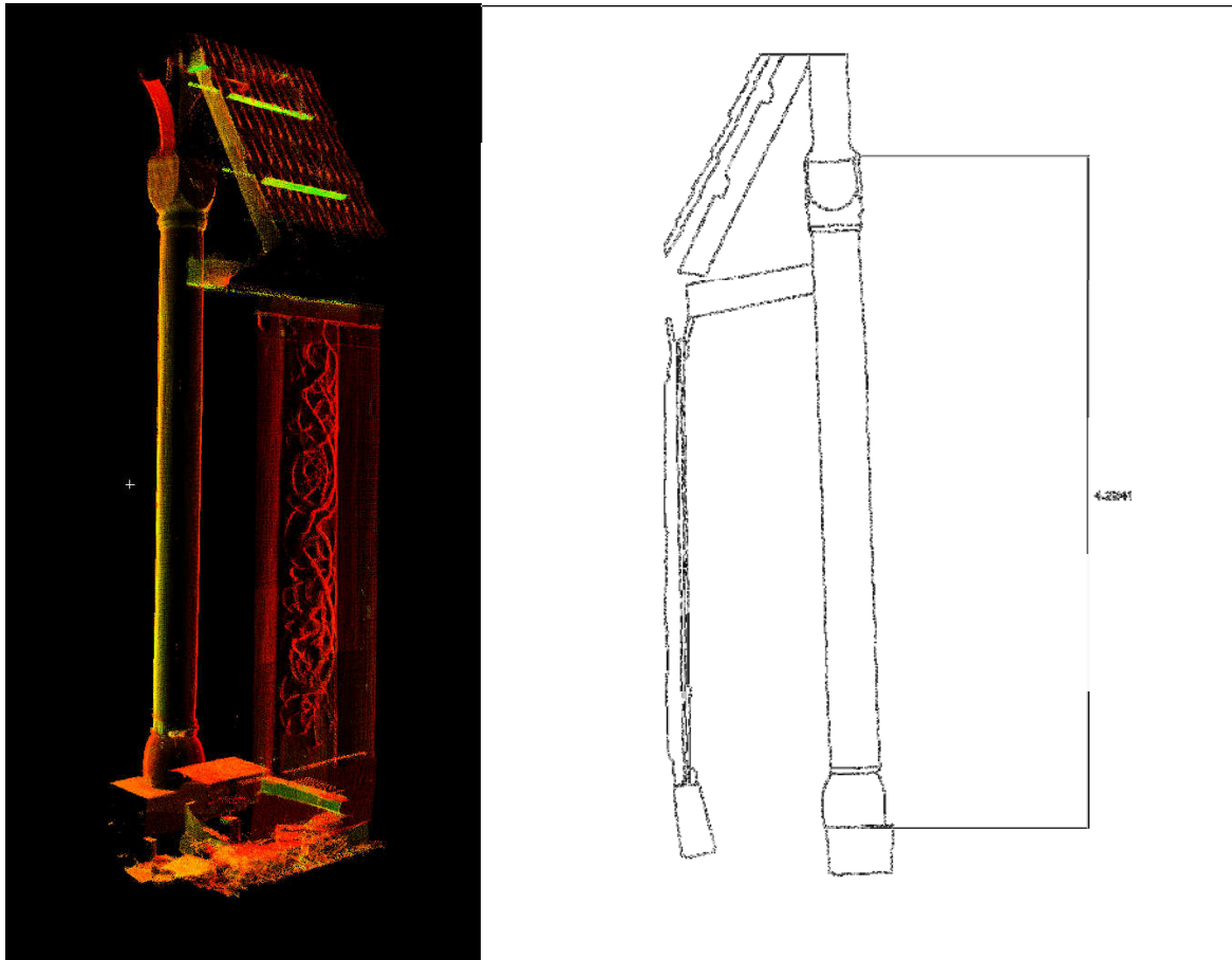
Figur 7 - Utsnitt fra nordveggen av kirken. Til venstre: Utsnitt fra punktssky. Til høyre: Strektegning av samme utsnitt med den nordre grunnsvillan ytterst til venstre. Legg merke til grunnsvillens posisjon i forhold til veggen.
